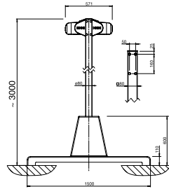
Betonsockel mit abgerundetem Design Basamento in cemento e design arrotondato
