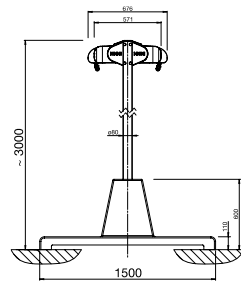
Betonsockel mit Volant-Plus Basamento in cemento e Volant-Plus
