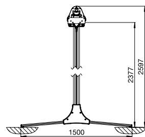
Querfuss Appoggio trasversale
